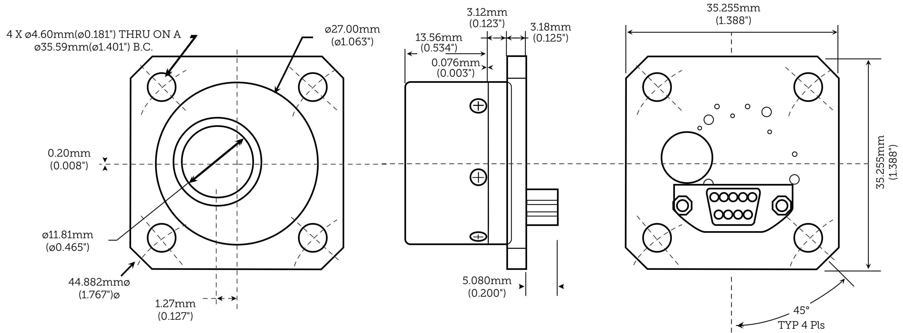
MK26-1 Dimensions
