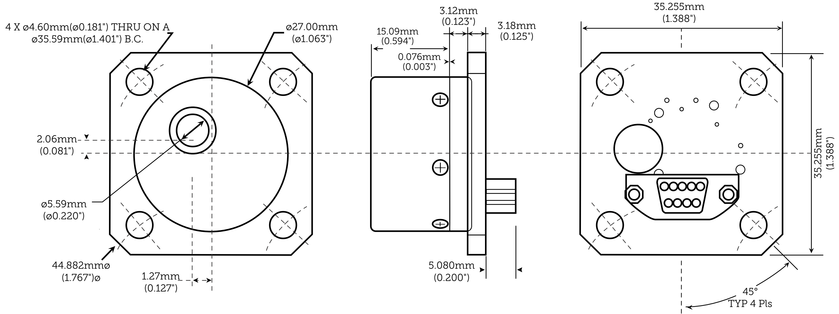
MK26-4 Dimensions
