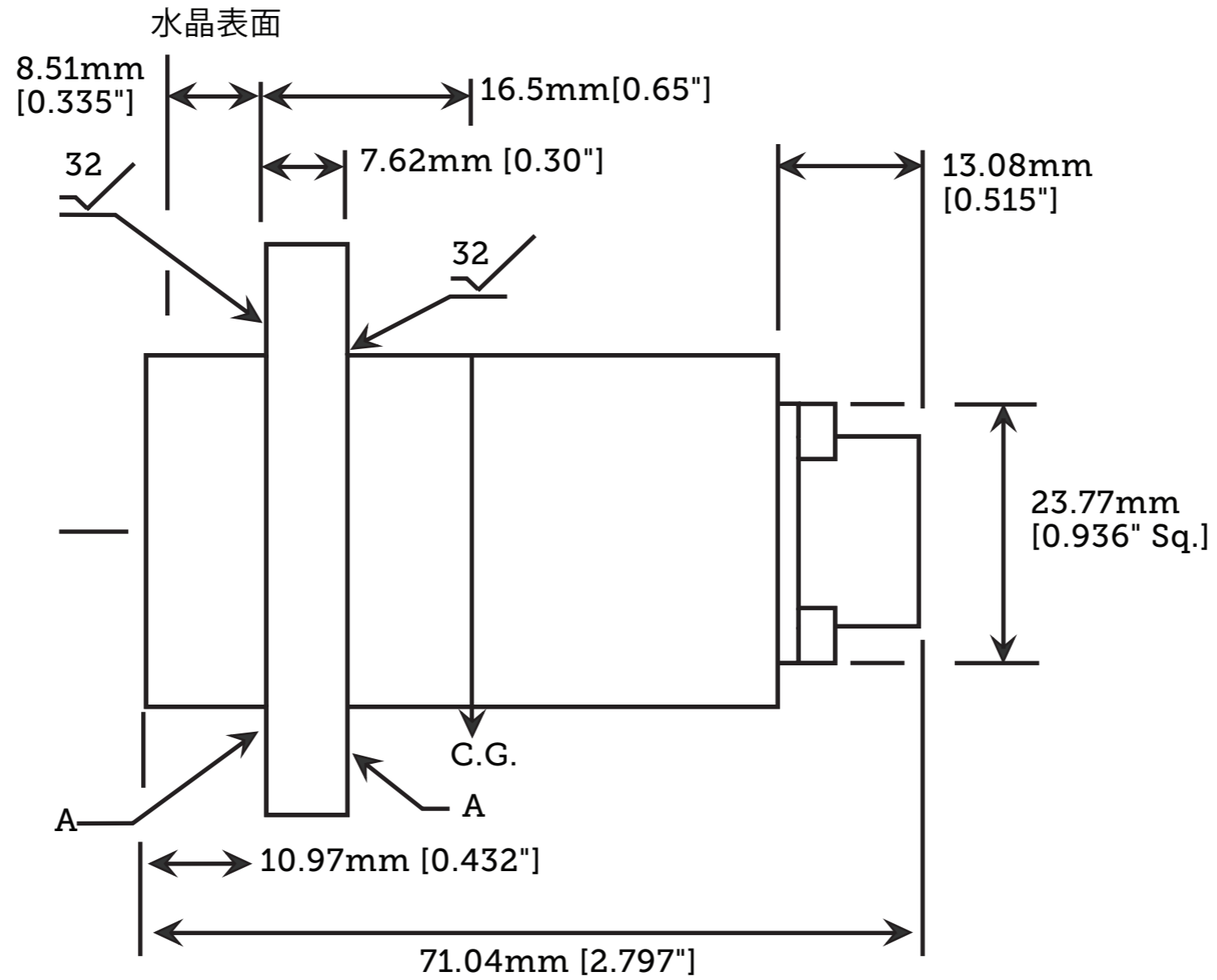
MK10の側面図
