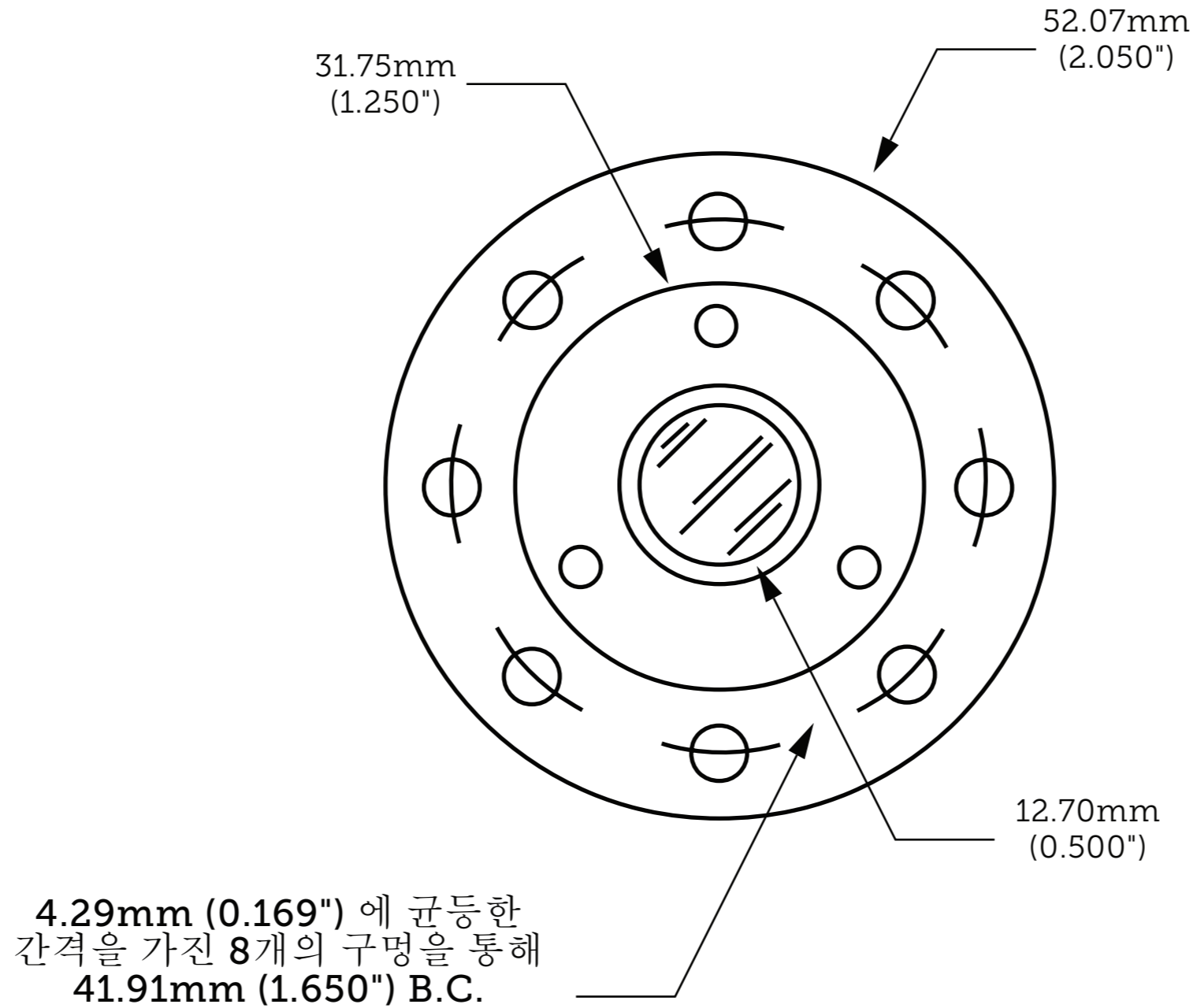
MK10 전면 다이어그램
