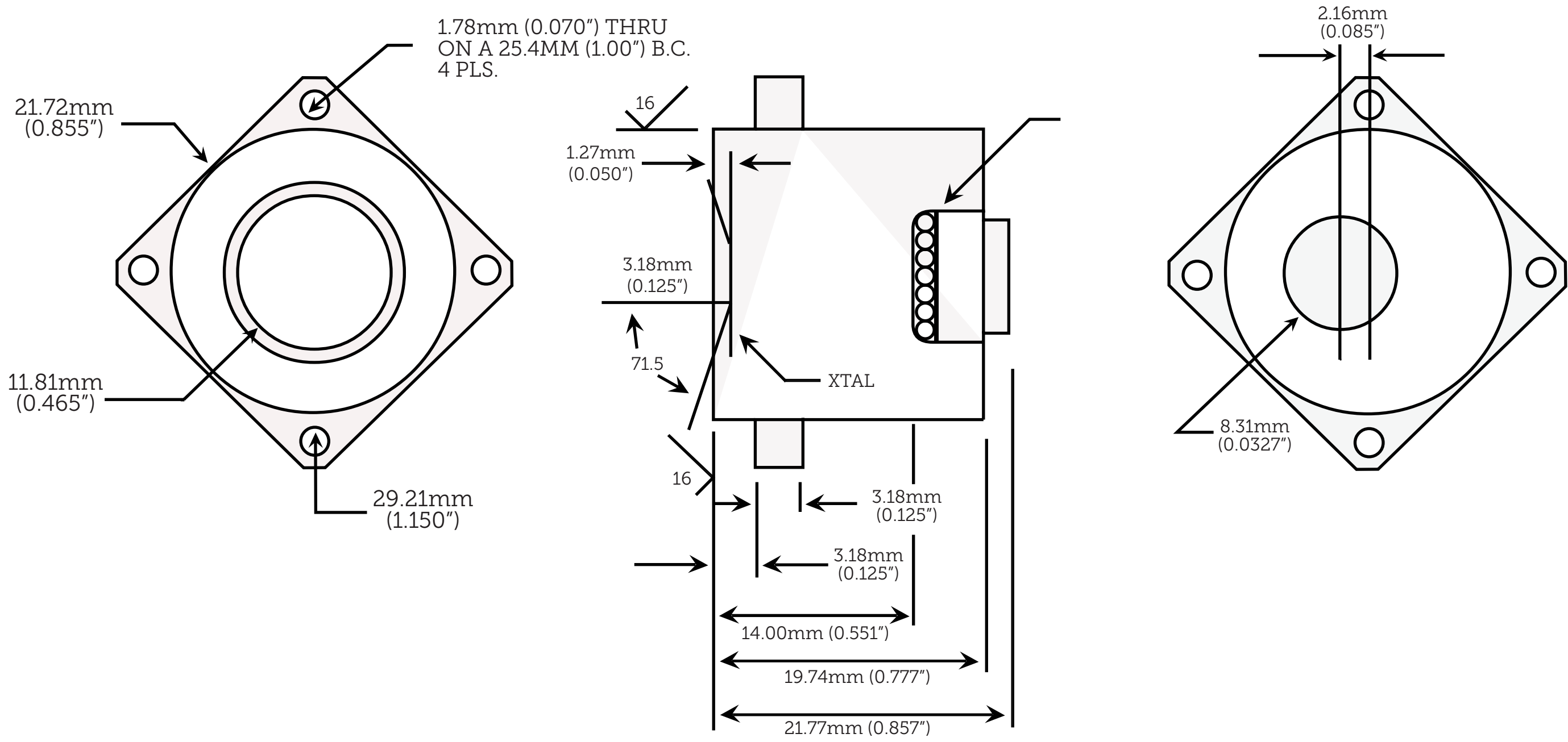
MK16 Abmessungen
