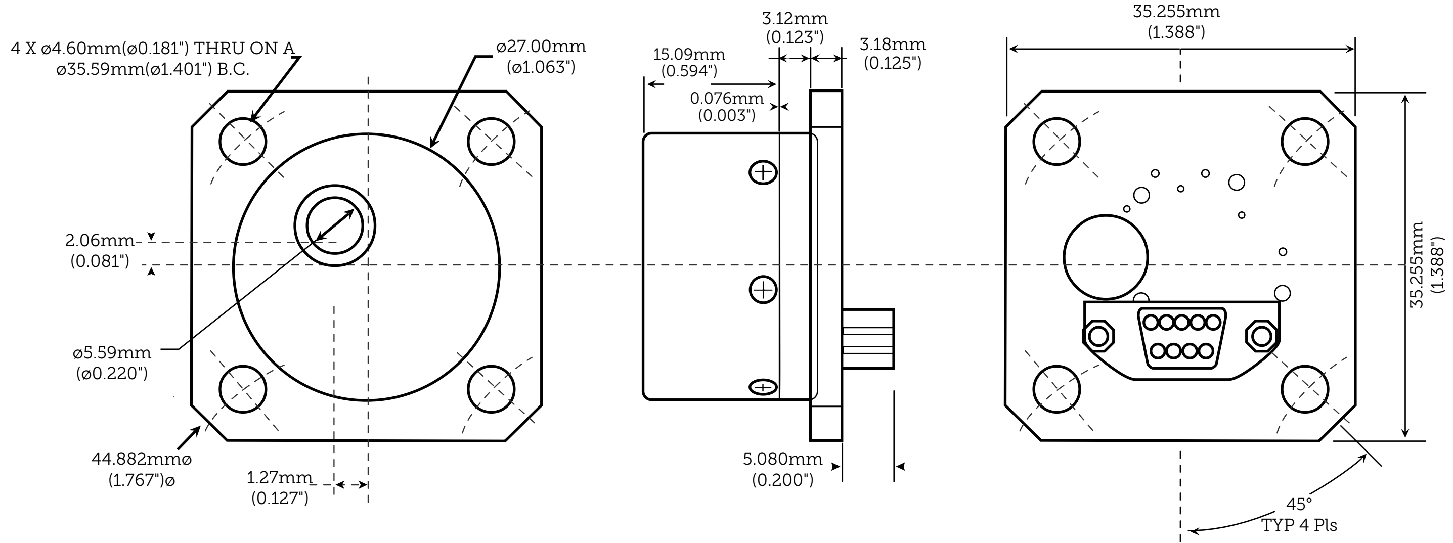
MK26-4 Abmessungen
