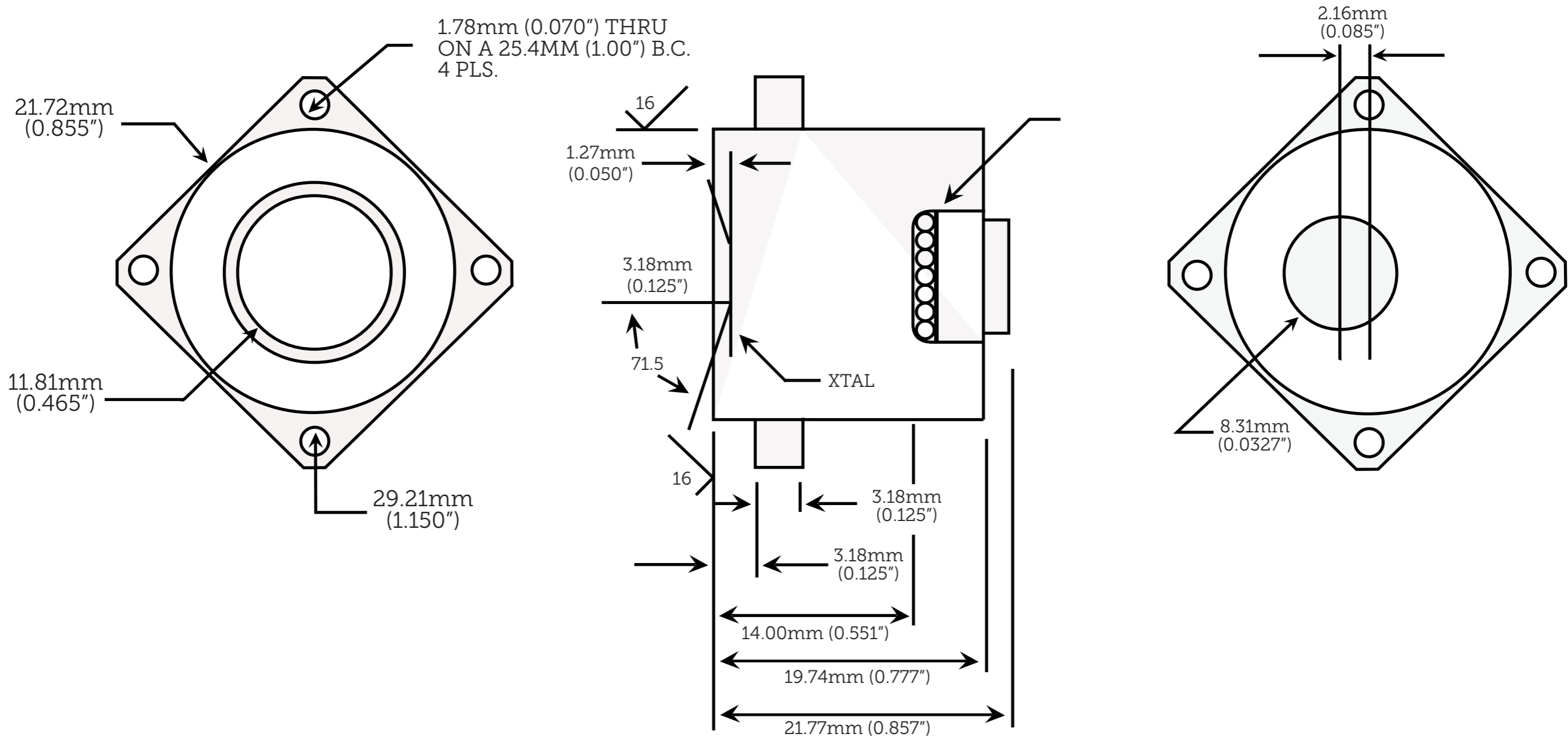
MK16 Dimensions
