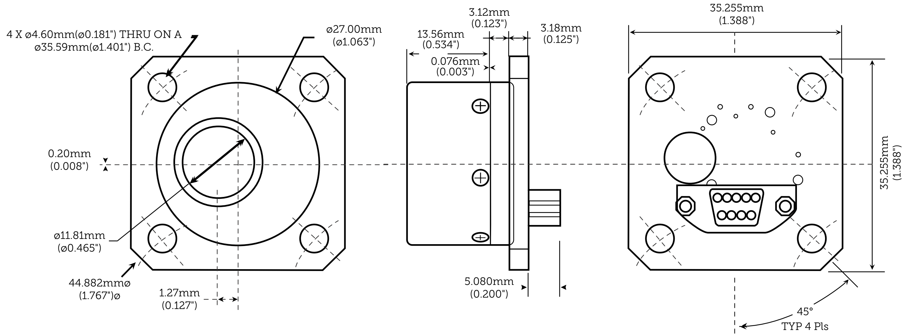
MK26-1 寸法
