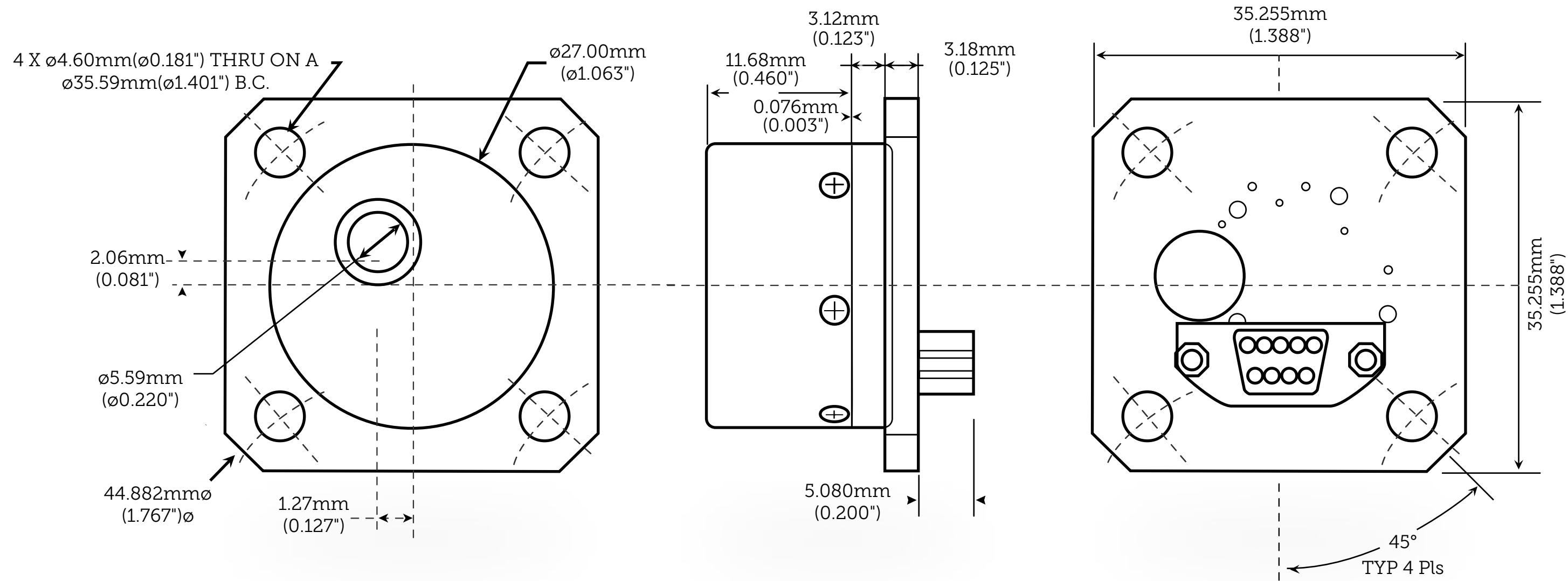
MK26-2 寸法
