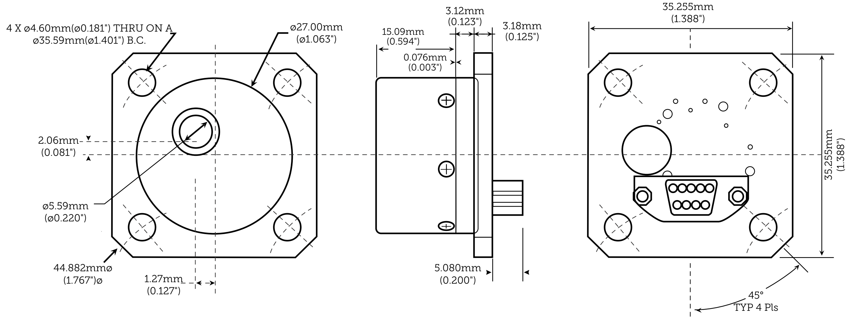
MK26-4 寸法
